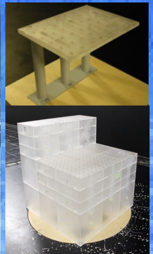
風洞実験模型
