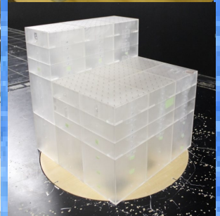
風洞実験模型
