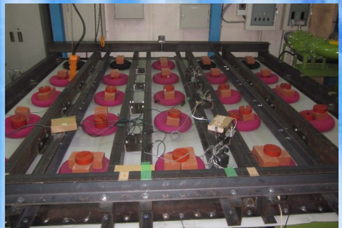
機械固定的工法防水システムの耐風圧性能試験
